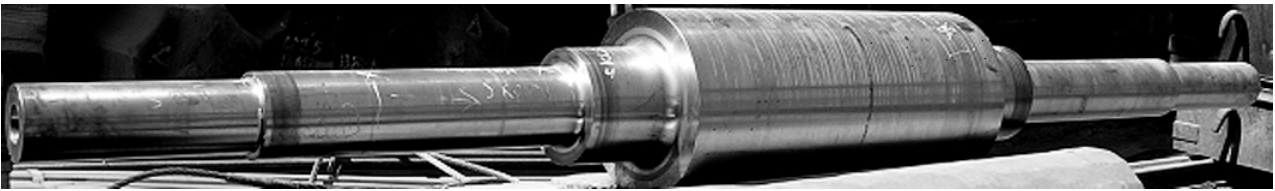
Figure 10: Defective generator rotor shaft – forging No. 447 660 Slika 10: Defektna gred rotorja generatorja – odkovek št. 447 660
