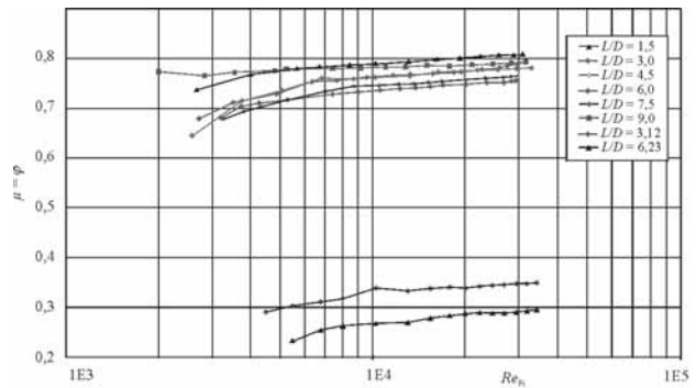
Figure 2: Dependence of the filter-outlet coefficient on the Reynolds number and the ceramic filters' slenderness Slika 2: Odvisnost izhodnega koeficienta od Reynoldsovega števila in od vitkosti filtra
