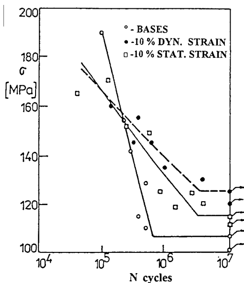
Figure 2: Woehler curves for a low carbon steel Slika 2: Wöhlerjeva krivulja za maloogljicno jeklo
