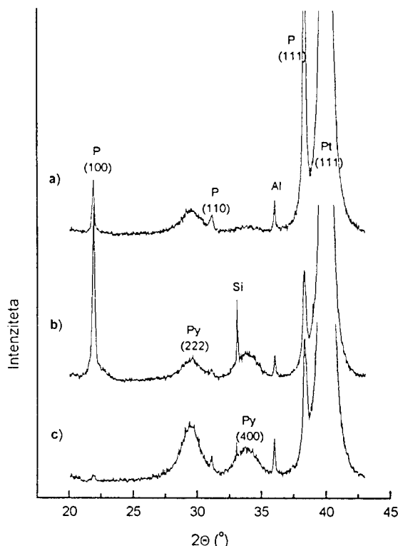
Slika 1: Rentgenski spektri plasti PLZT na a) kristalinični plasti PT, b) amorfni plasti PT in c) TiO 2 /Pt/TiO 2 /SiO 2 /Si (podlagi I) po segrevanju na 500°C, 10 minut (P-perovskitna faza, Py-piroklorna faza, Al-aluminijasti nosilec)
